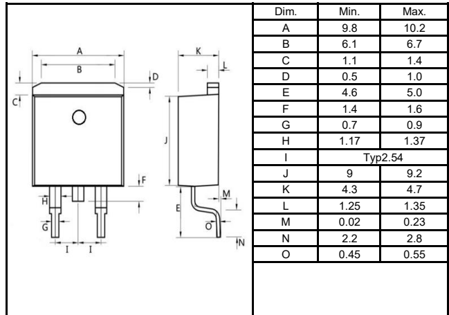
T0-263C
